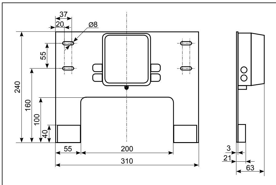
Рисунок 7. Габаритные и установочные размеры
